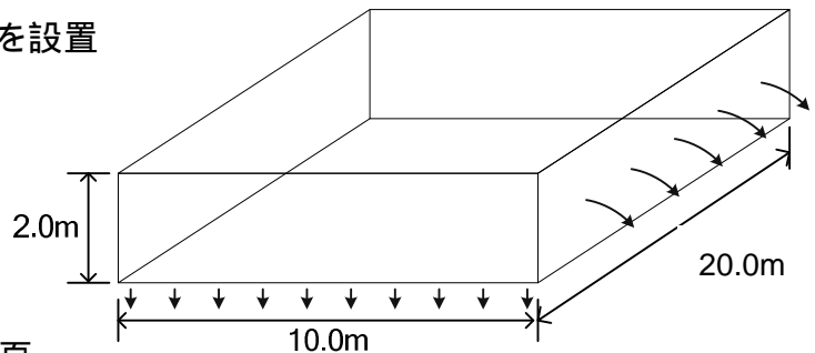
公園等に設置する場合の 地下貯留浸透施設構造図
