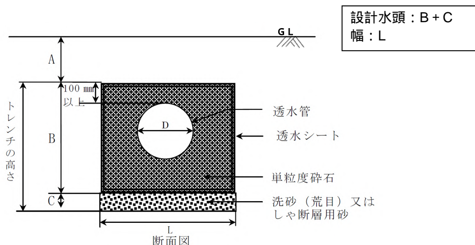
図 4.7 浸透トレンチの構造
