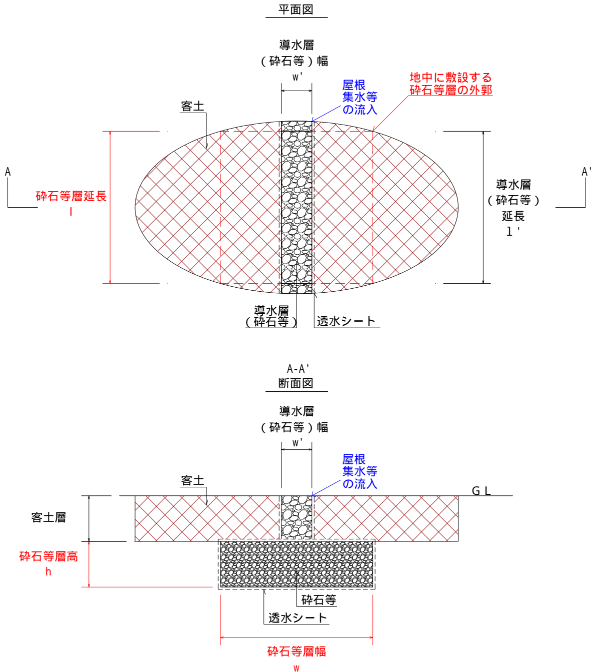
図 4.11 客土部分が楕円(砕石等層の形状は正方形や矩形)の雨庭のイメージ図
