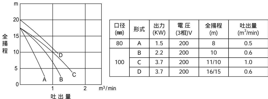
図 4.71 ポンプの性能曲線と仕様
