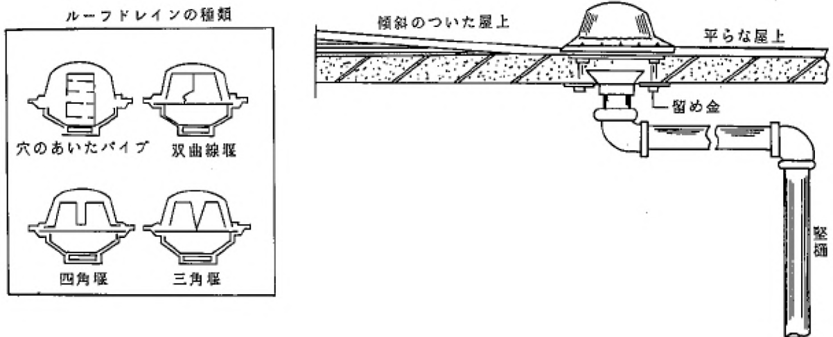
図 4.2.2 ルーフドレインの例
