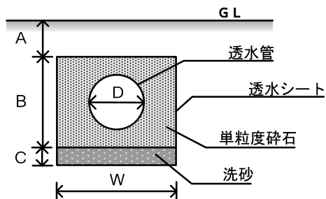
【断面図】
