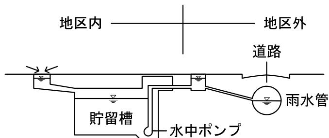
図 4.19 地下式貯留施設構造概念
