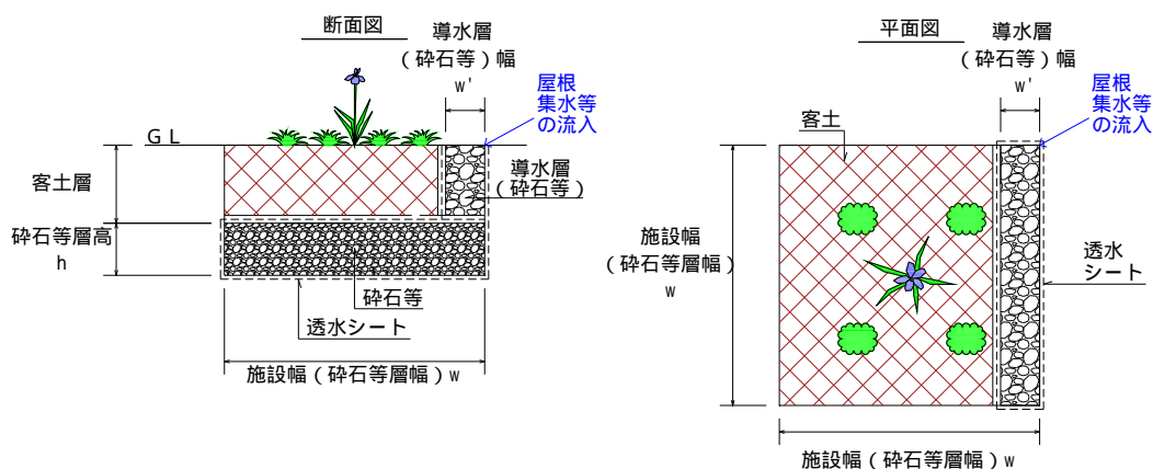
図 4.47 雨庭(覆土植栽型)の標準的構造
