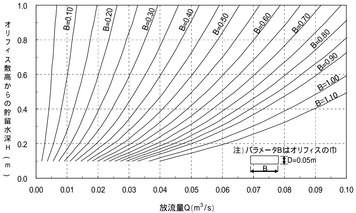
図 4.66 オリフィス水深 H ~ 放流量 Q 関係図 (D = 0.05 m)
