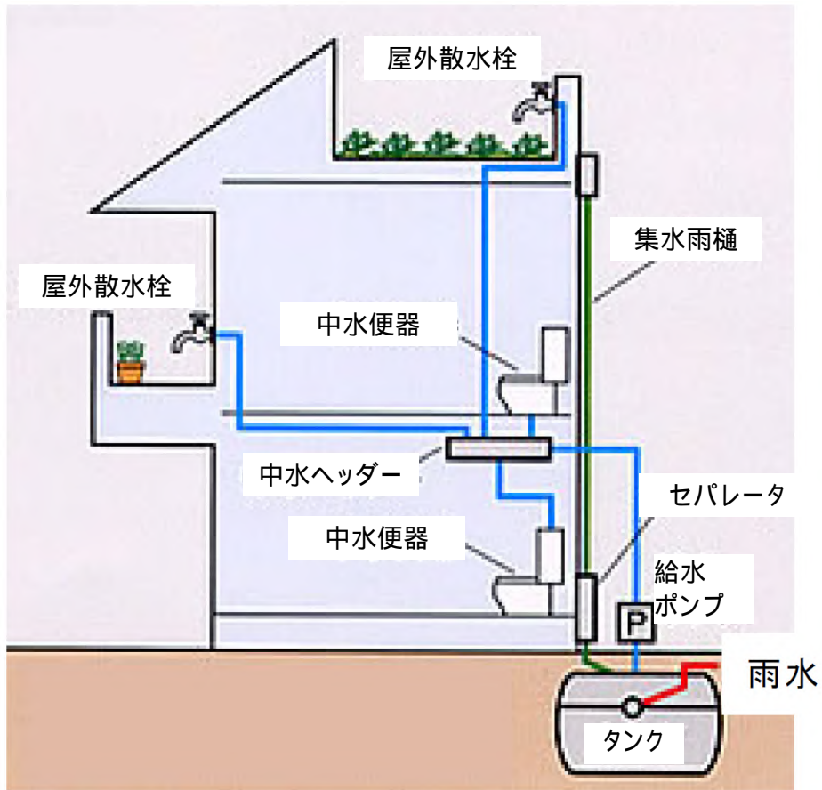
図 4.25 中水利用例
