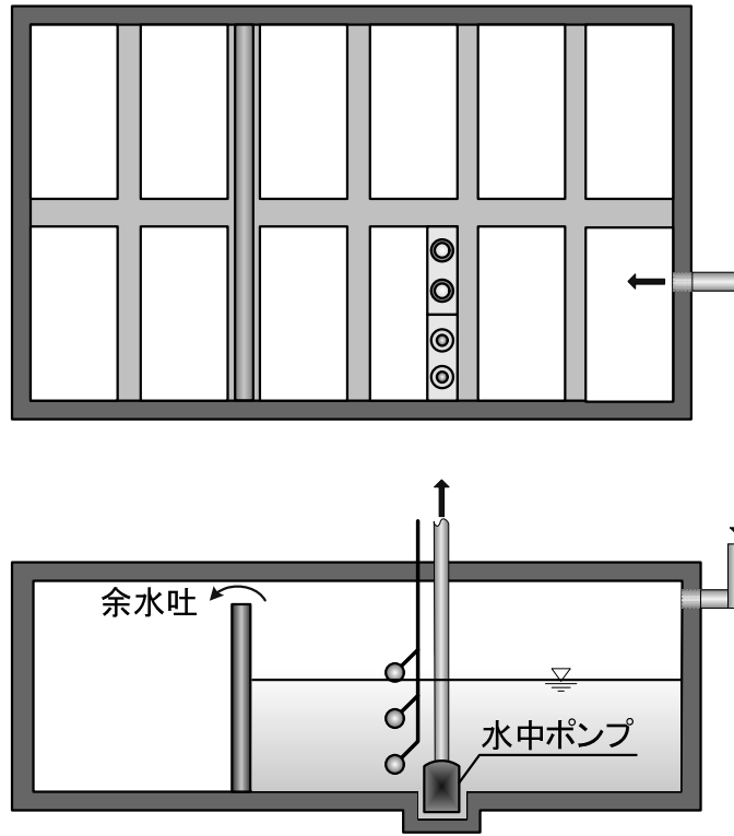
図 4.21 貯留槽と水中ポンプ
