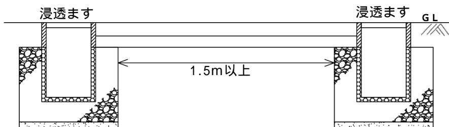
図 4.26 浸透施設間の距離
