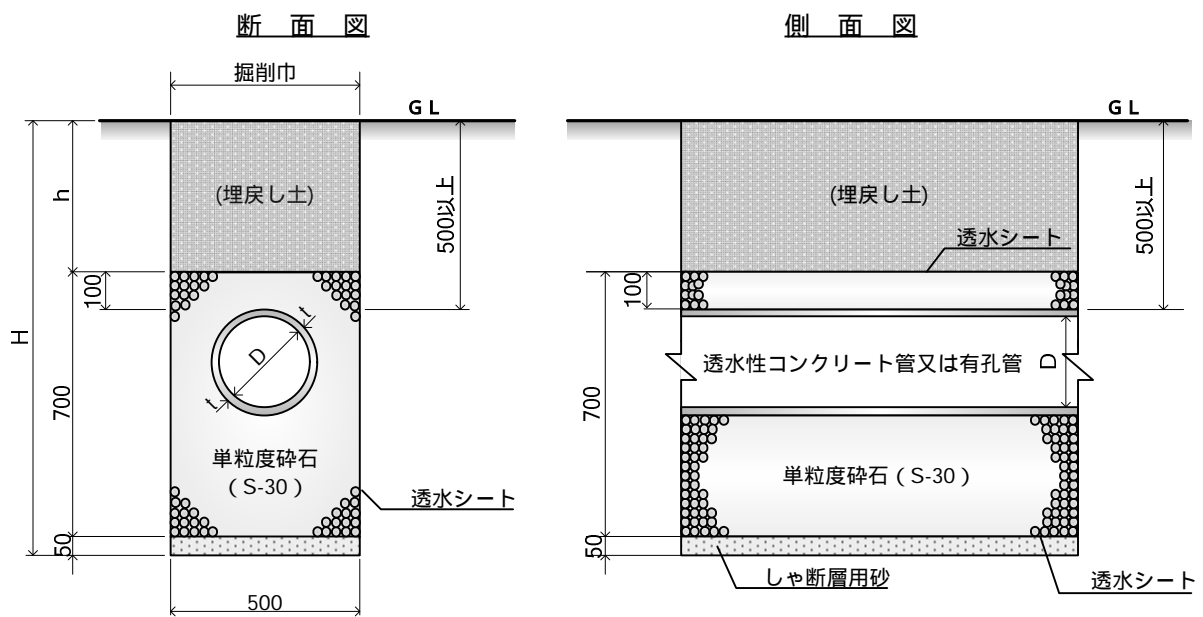
図 4.35 地下透水管( 型)(500×700)(世田谷区標準構造図集より)
