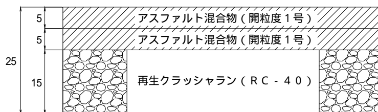
図 4.36 透水性舗装 35 型(車道用) (世田谷区標準構造図集より)
