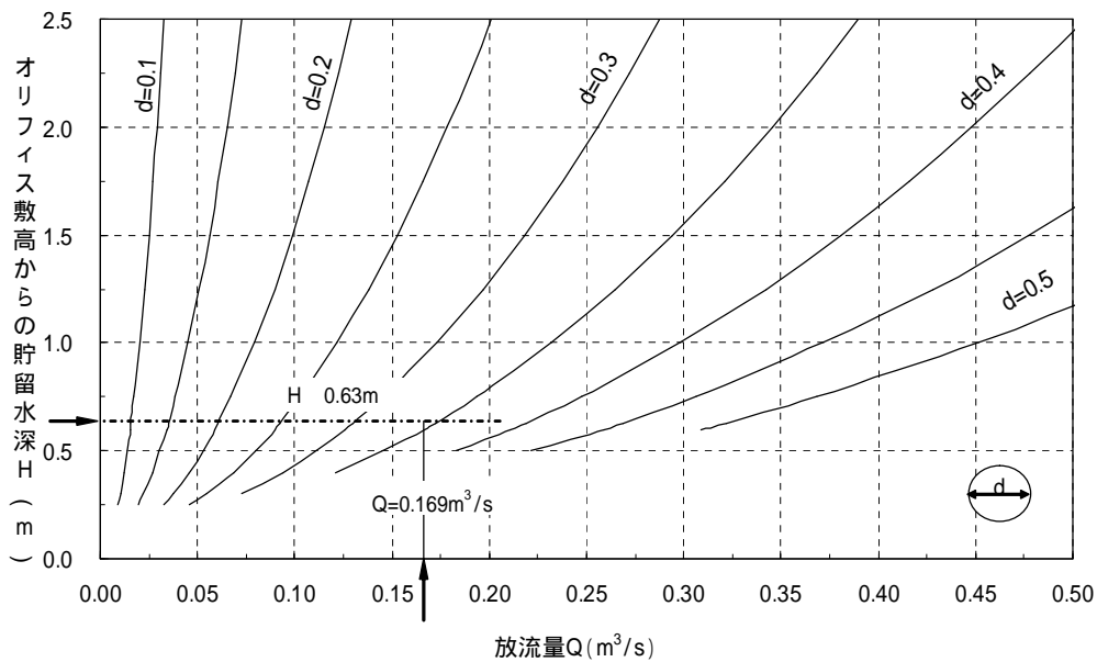
図 4.70 オリフイス水深 H ~ 放流量 Q 関係図(円形)
