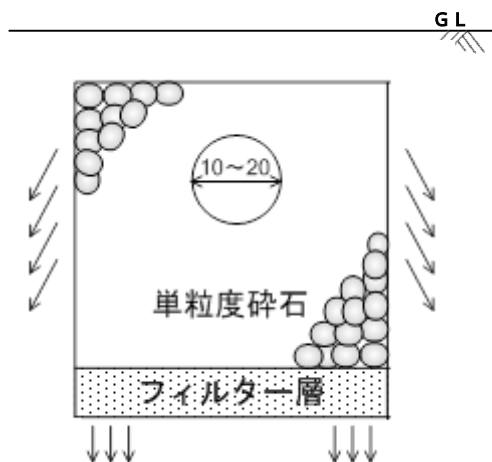
図 4.32 浸透トレンチの例
