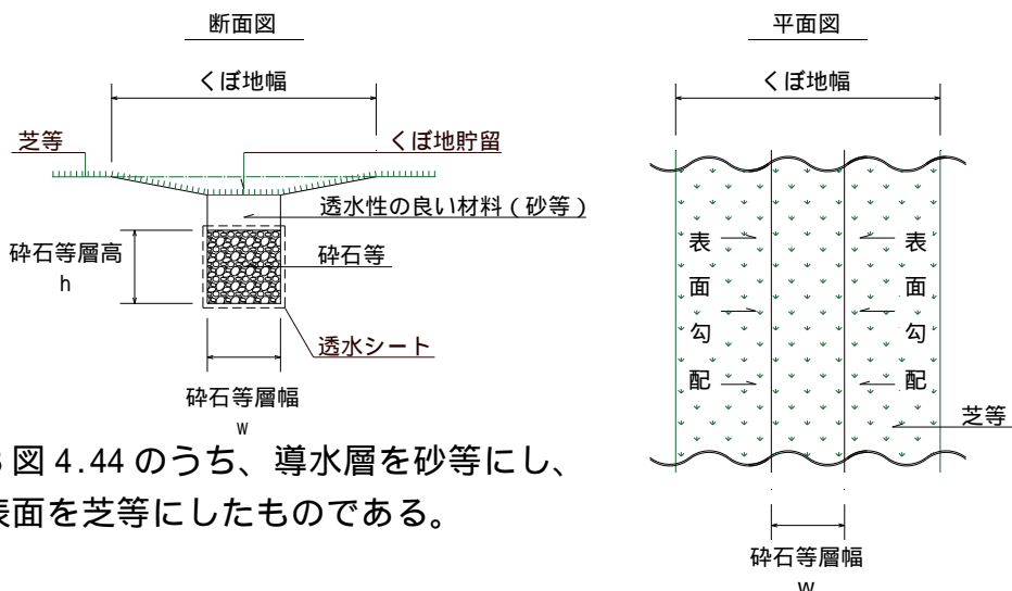
図 4.54 トラフアンド緑溝（芝張側溝 + 緑溝）
