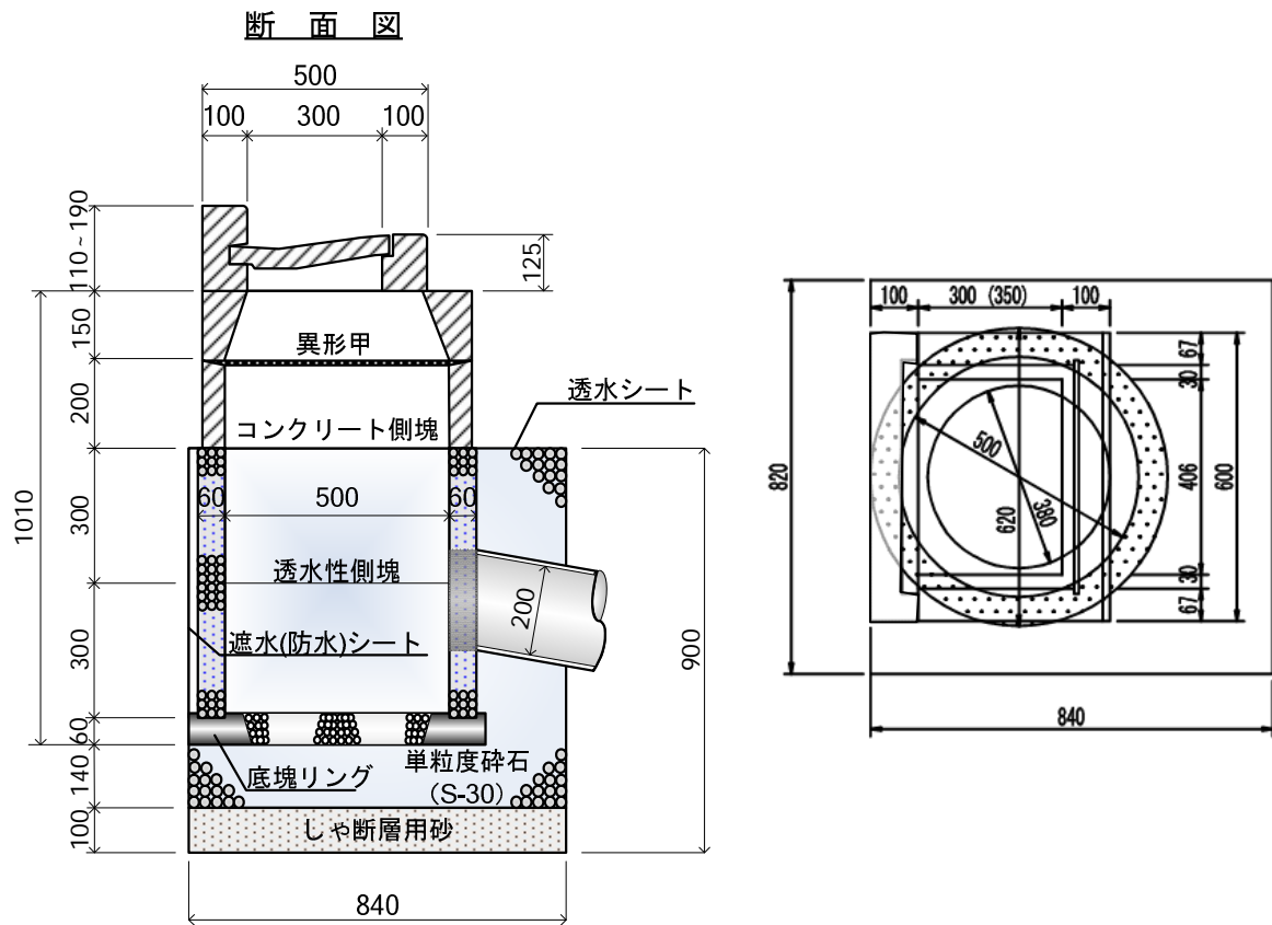
図 4.39 L形用浸透ます( 500)(H=1000)(世田谷区標準構造図集より)
