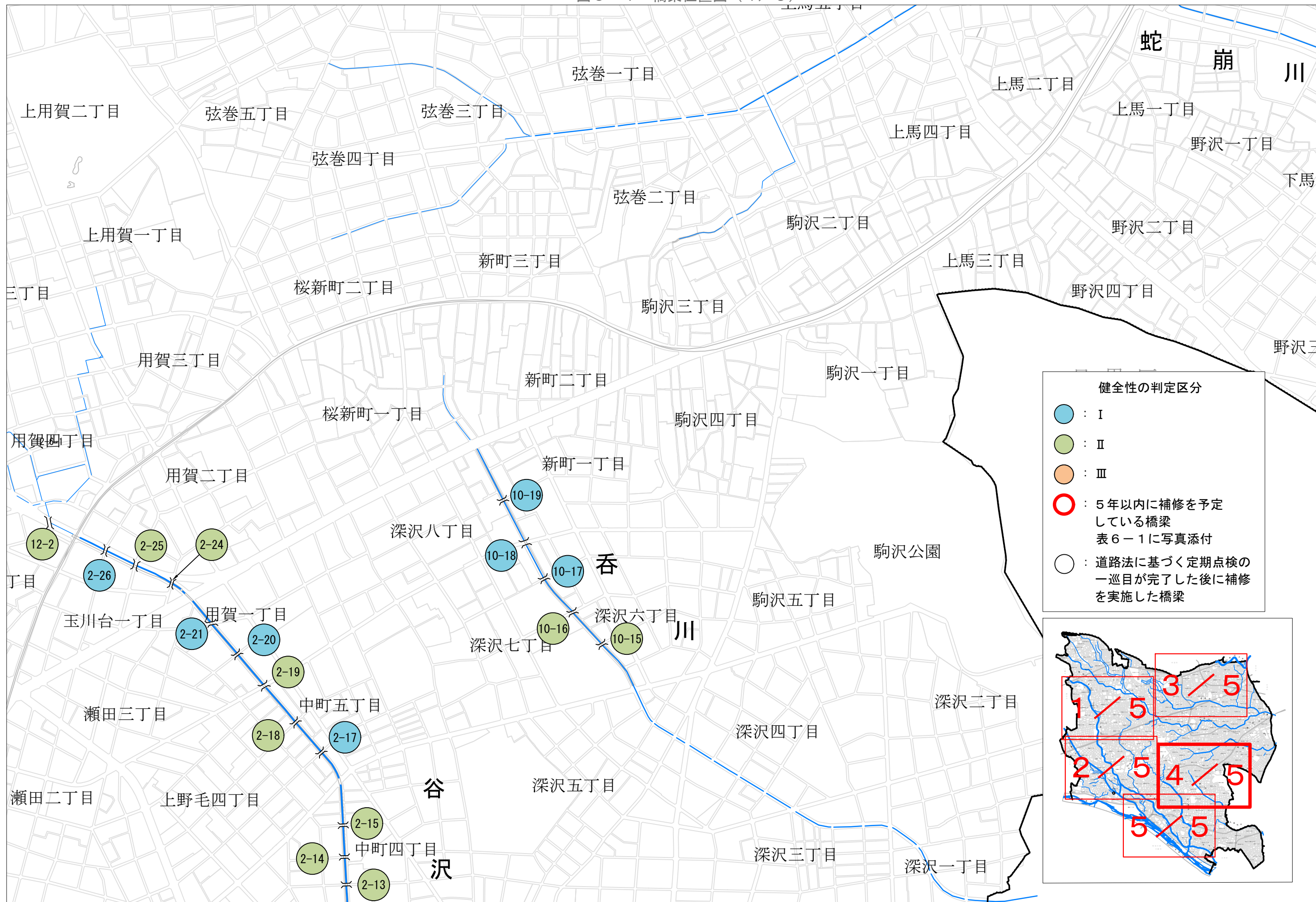
図6-1 橋梁位置図(4/5)
