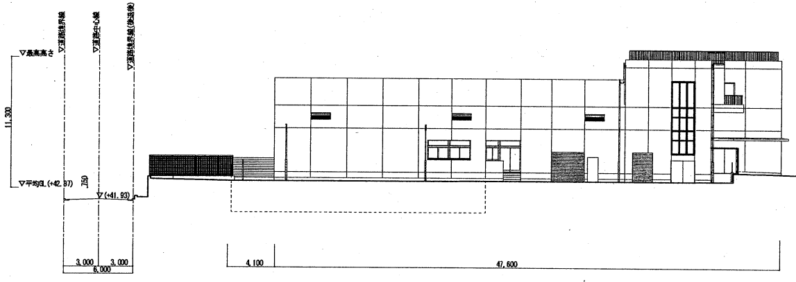
複合施設棟 西側立面図
