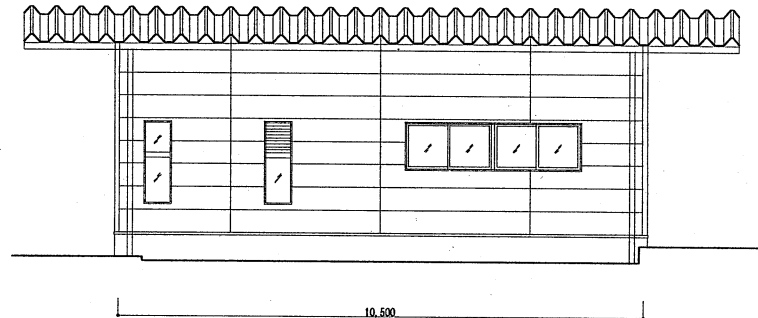
付属棟 東側立面図
