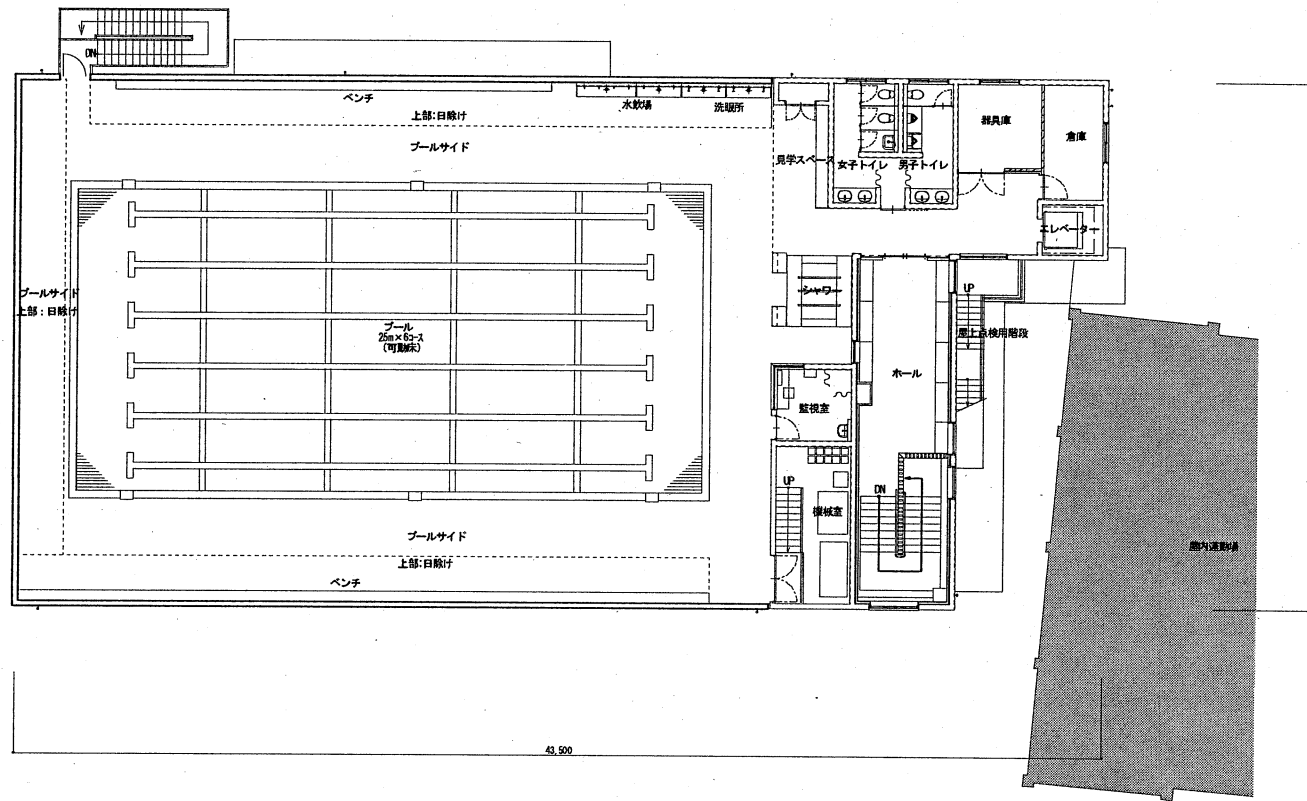
2階平面図
