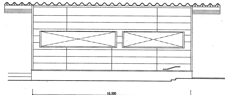
付属棟 西側立面図
