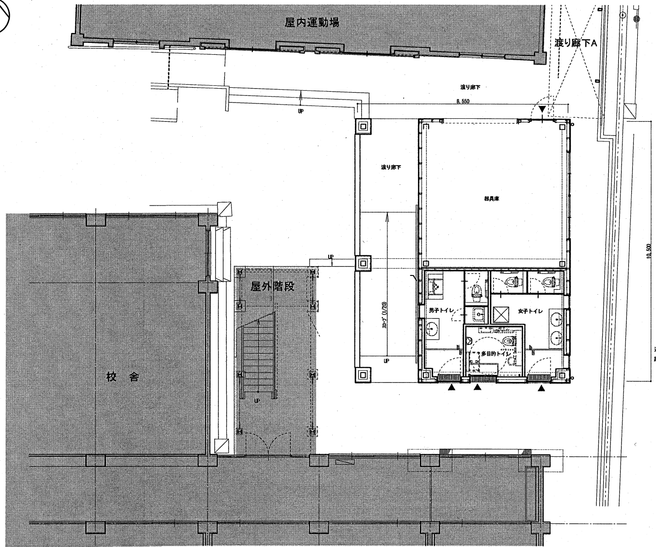
付属棟 平面図
