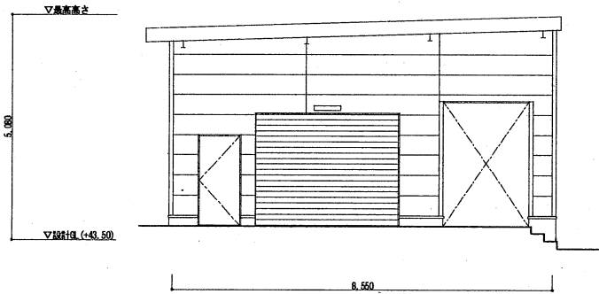
付属棟 北側立面図
