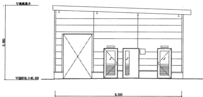
付属棟 南側立面図
