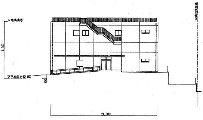
複合施設棟 南側立面図
