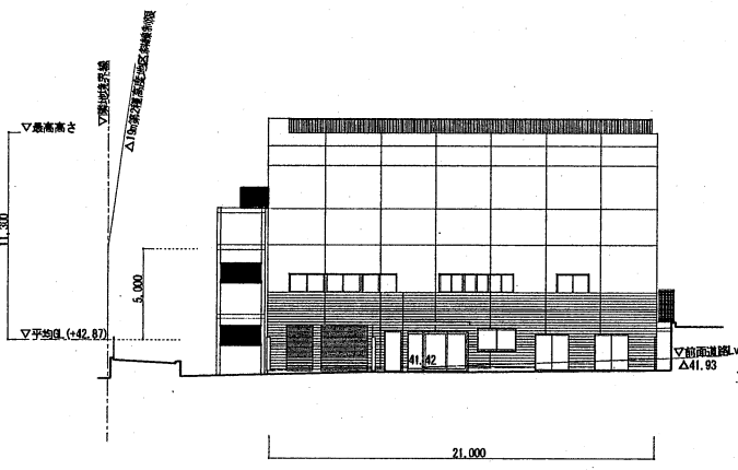
複合施設棟 北側立面図
