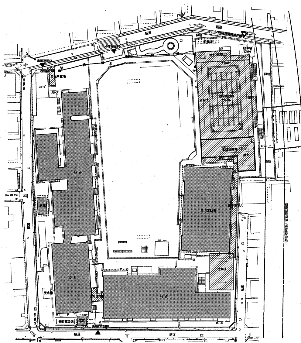
配置図
