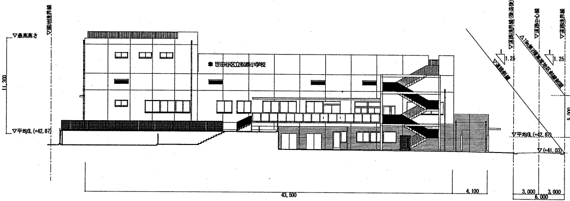
複合施設棟 東側立面図
