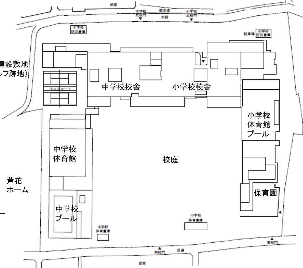
芦花小学校 芦花中学校 既存配置図
