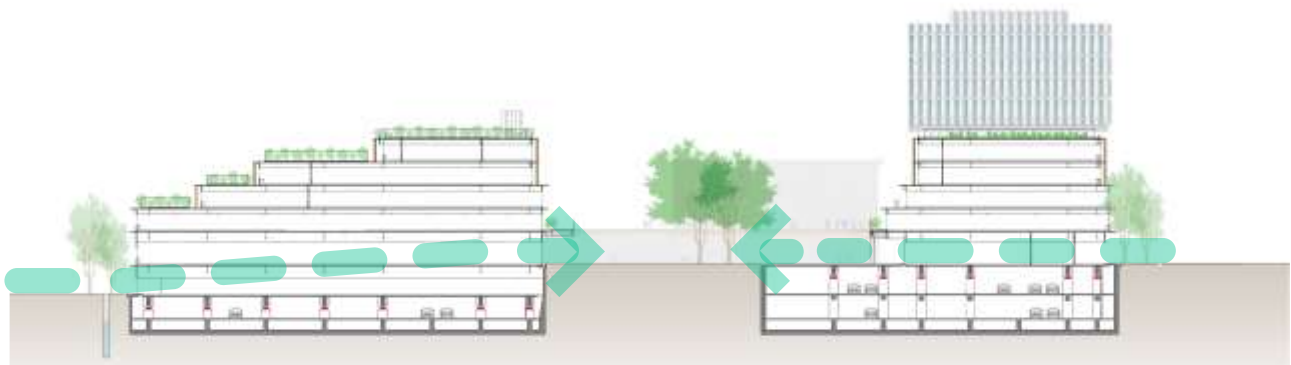
断面図兼立面図
