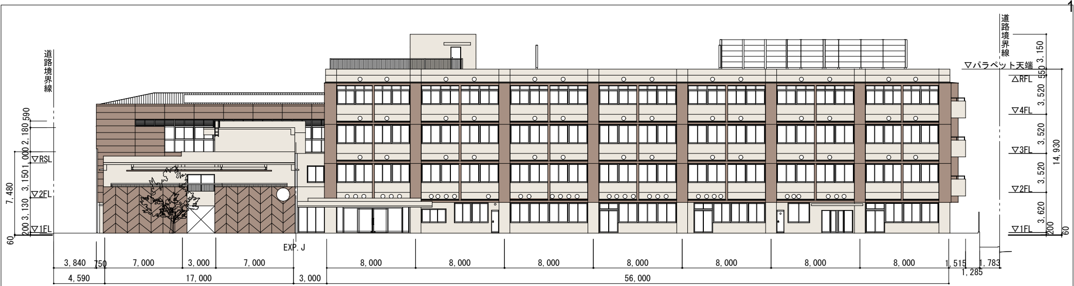
南側立面図
