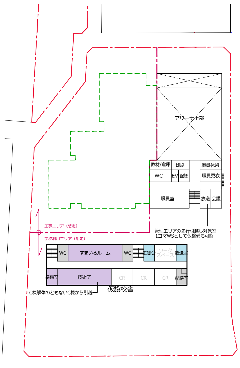
<2階>
