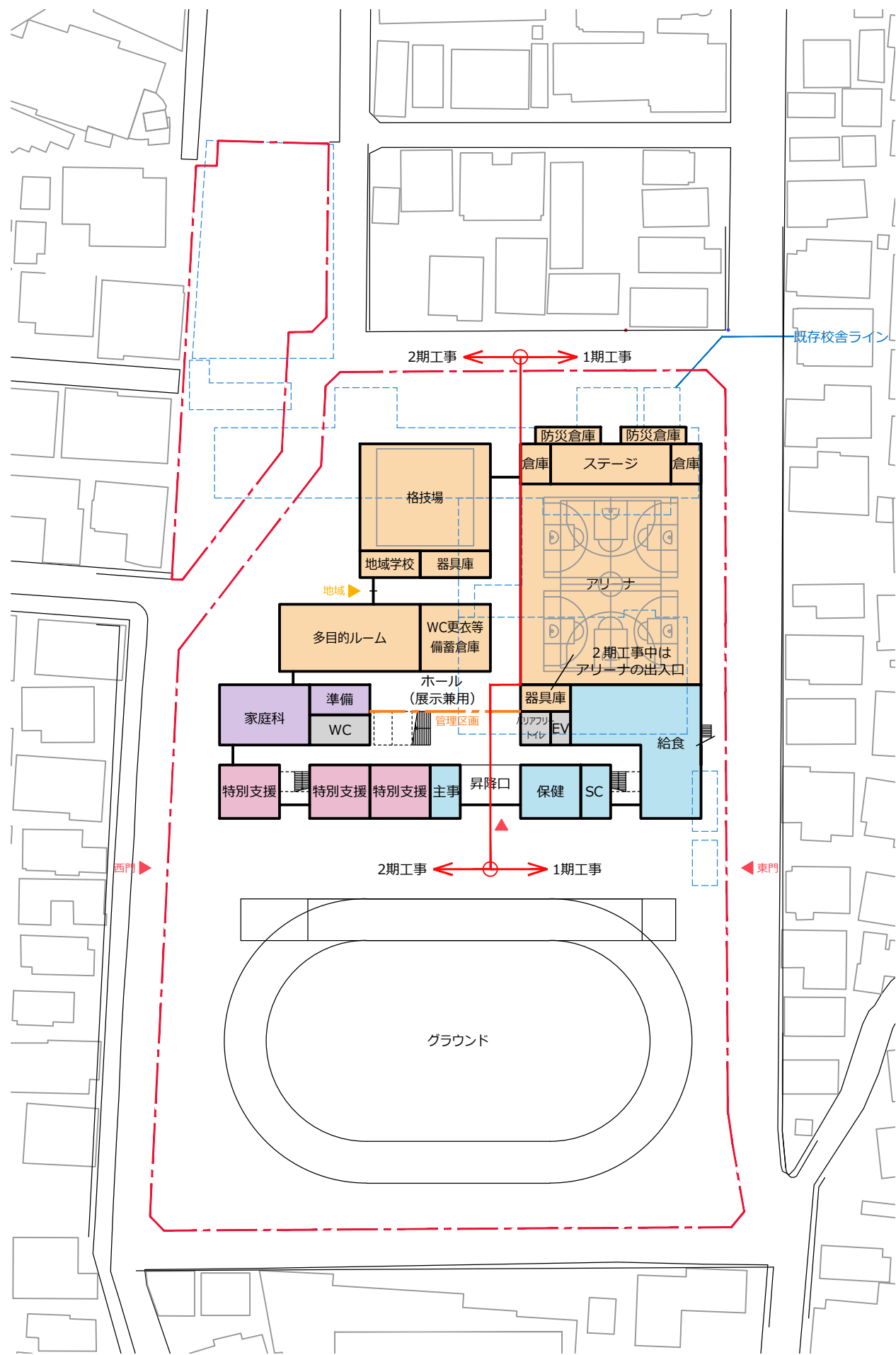
<配置図兼1階>
