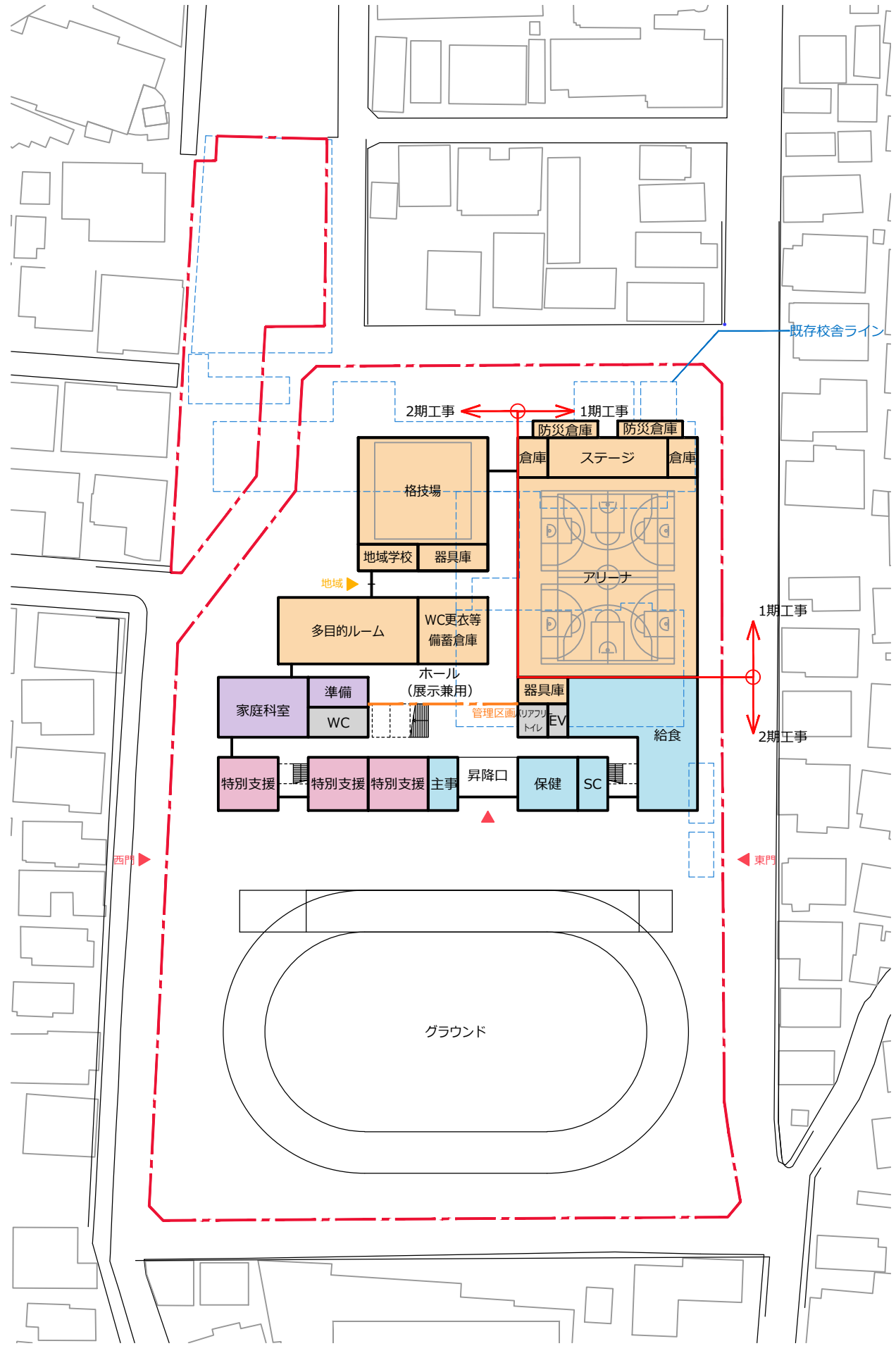
<配置図兼1階>
