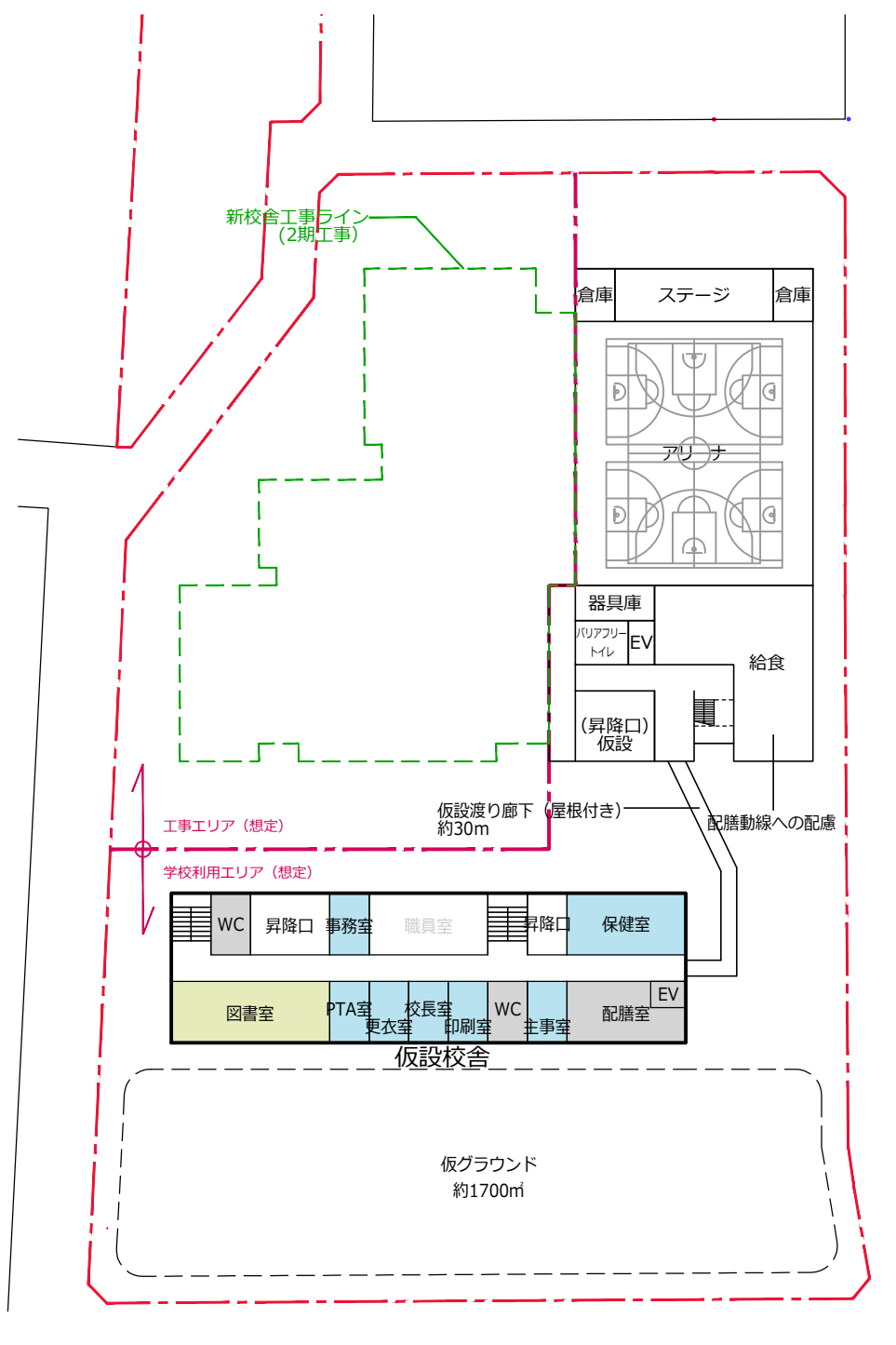
<1階>
