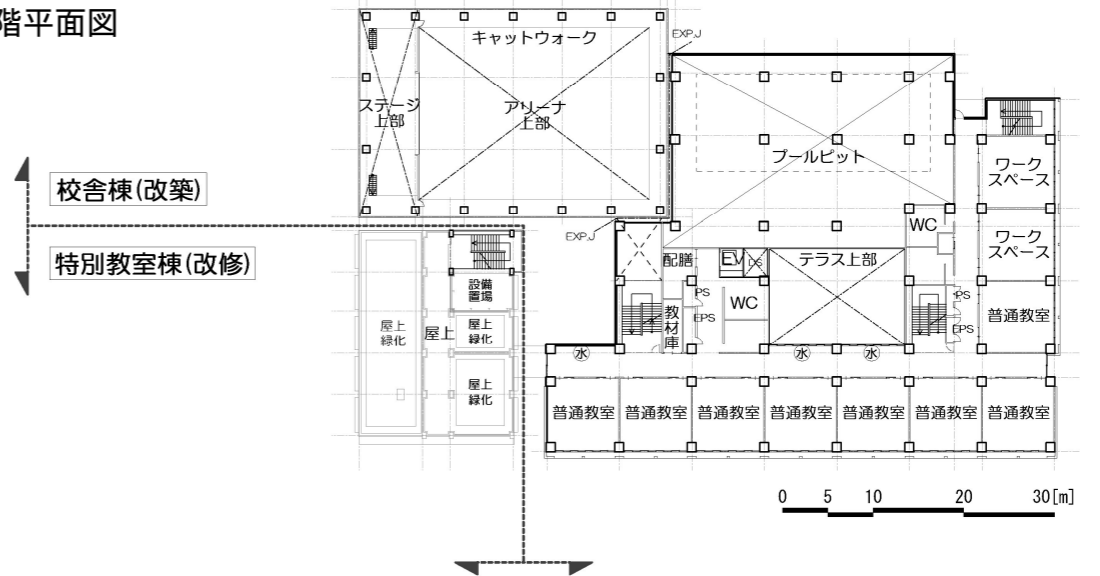
○4階平面図 (
