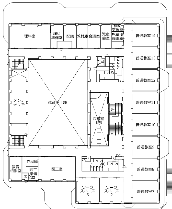
3階平面図
