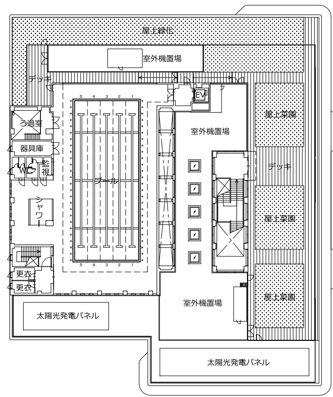
4階平面図
