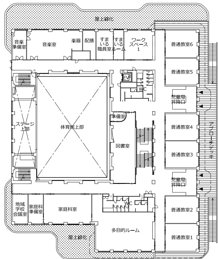
2階平面図
