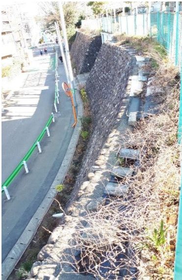
現況写真①：西側玉石擁壁
