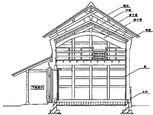
図1 旧浦野家住宅土蔵・断面図
