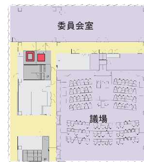
9階平面図
