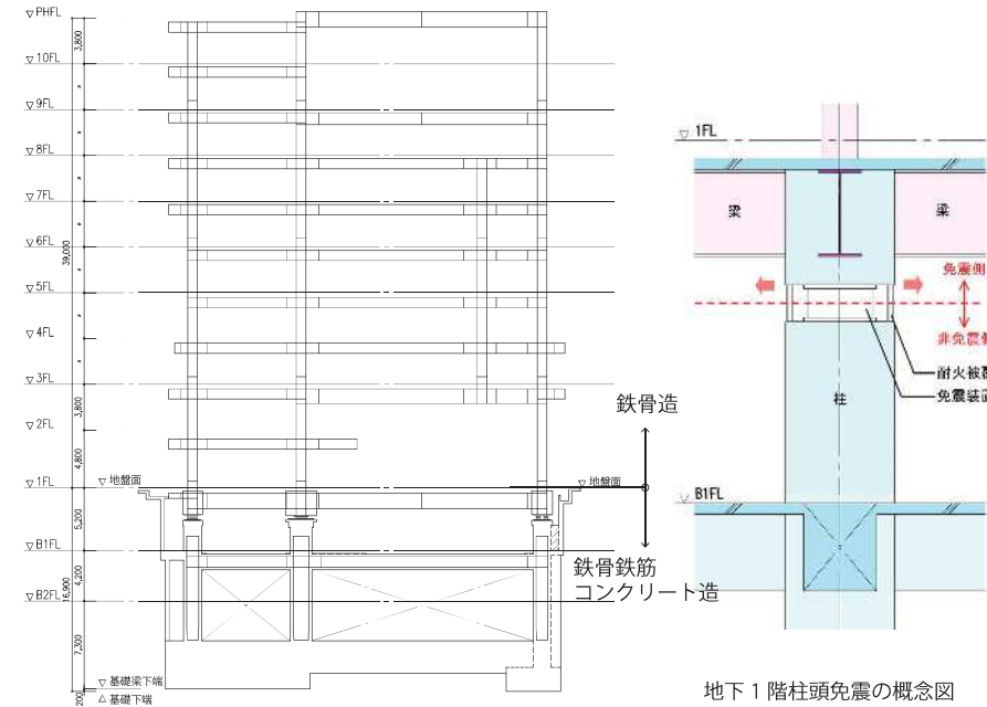
軸組図（東棟）
