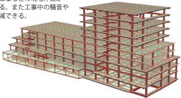
上部構造の架構モデル図（東棟）
