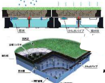
屋上緑化貯留のイメージ
