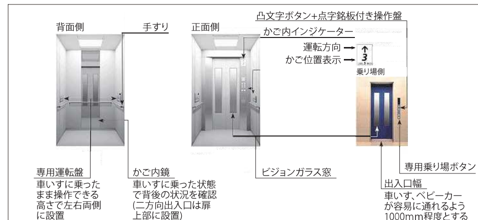
車いす対応仕様のエレベーター乗り場、かご内イメージ
