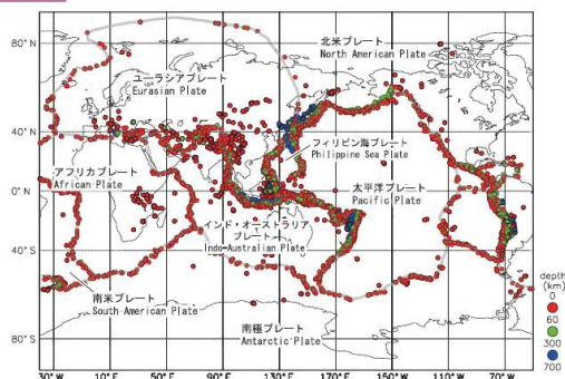
図1-1-2 世界の震源分布とプレート
