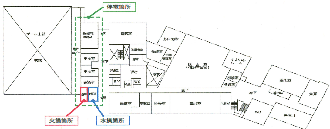
1階平面図
