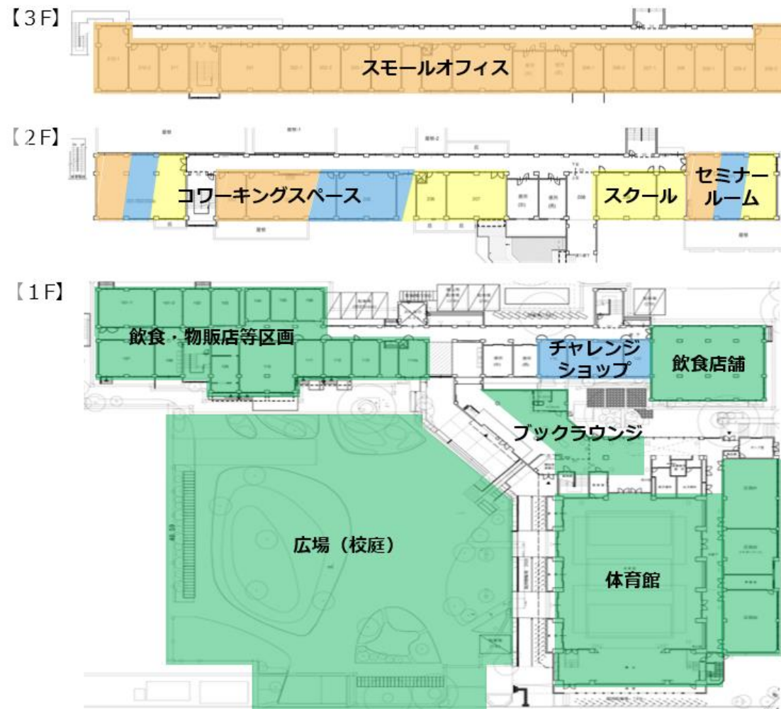
<施設平面図>
