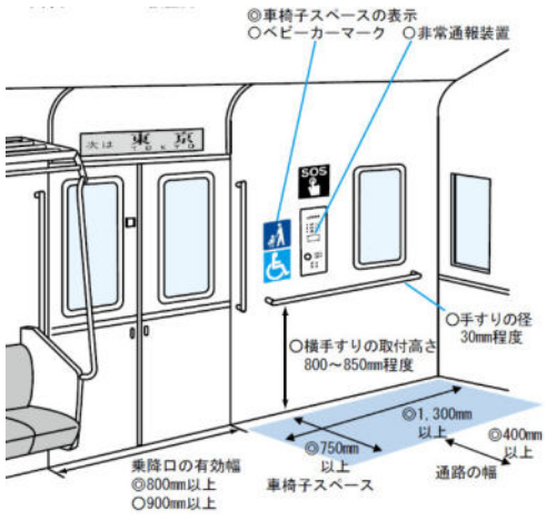
図 97 鉄道車両車いすスペースの設置例
