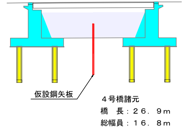
橋台断面図
