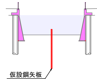
護岸断面図
